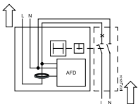
5SM6011-1
